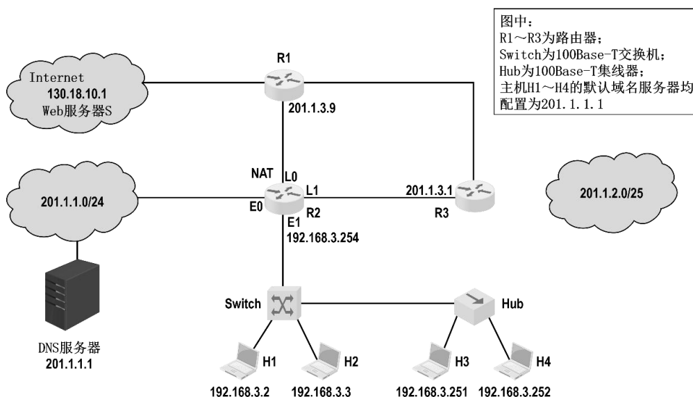
图 3-90 习题 3-77 的图
