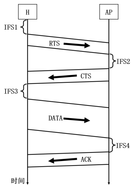
图 3-93 习题 3-86 的图
